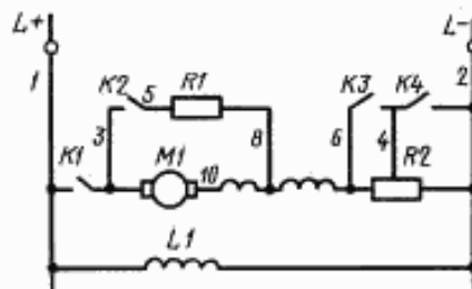
Черт. 8
